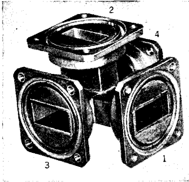
FIG. 18-6.—Magic T.
